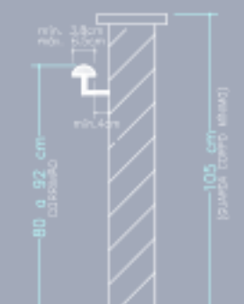
DETALHE DO GUARDA CORPO METÁLICO SEM ESCALA
