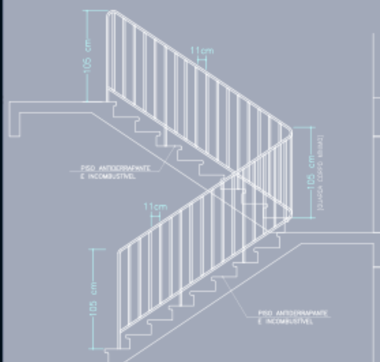
DETALHE DO GUARDA CORPO DA ESCADA SEM ESCALA
