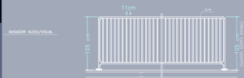
DETALHE DO GUARDA CORPO METÁLICO SEM ESCALA
